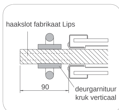
deur steekt 90 mm uit
