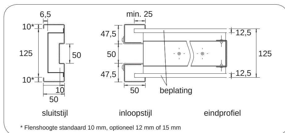
horizontale doorsnede SIW1, SIW2 en SIW10 bij muurdikte 125 mm
