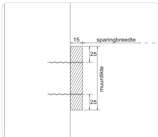
haakse wandaansluiting enkele schuifdeur in de wand
