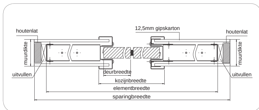
horizontale doorsnede SIW Electric
