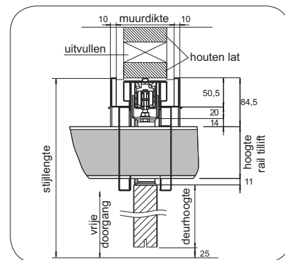
verticale doorsnede SIW-C1
