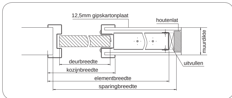
horizontale doorsnede SIW-C1
