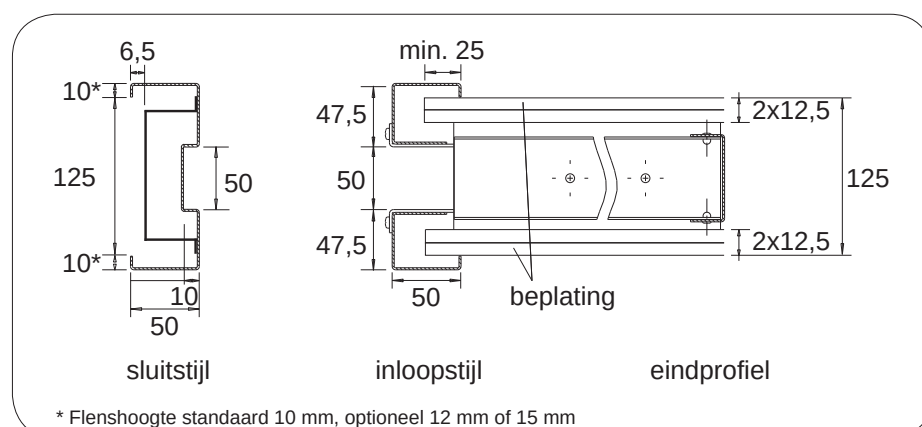
horizontale doorsnede SIW1, SIW2 en SIW10 bij muurdikte 125 mm, kast met dubbele beplating
