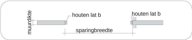
horizontale doorsnede
