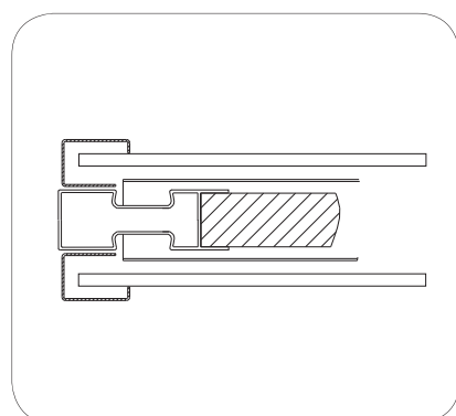
deur verdwijnt volledig in de wand
