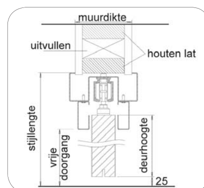
verticale doorsnede SIW1-30
