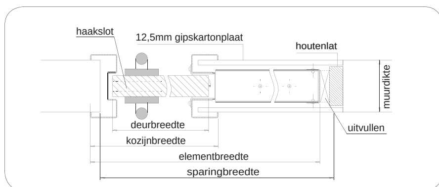
horizontale doorsnede SIW1-30
